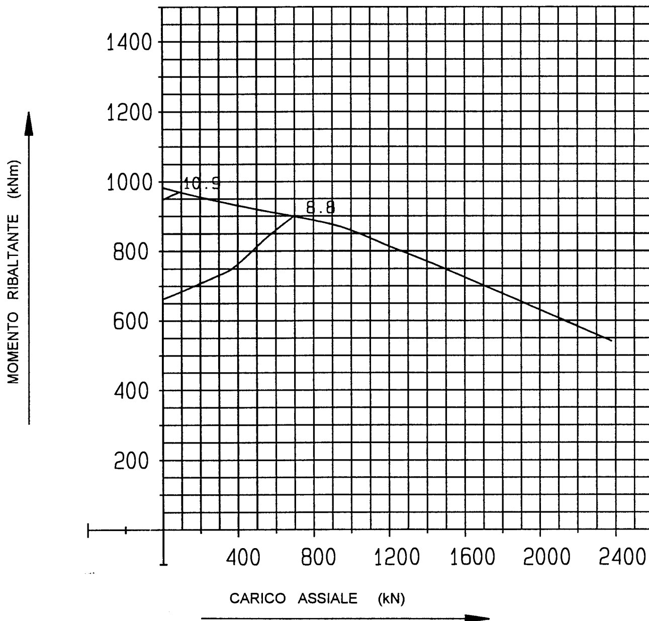
CURVE LIMITE RIFERITE A N°48 BULLONI GRANDEZZA M 22
