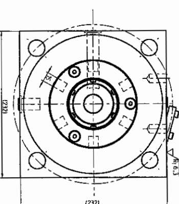
Ansicht X
