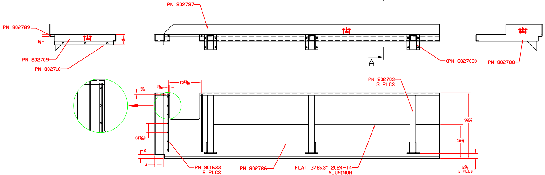
SECTION A-A
