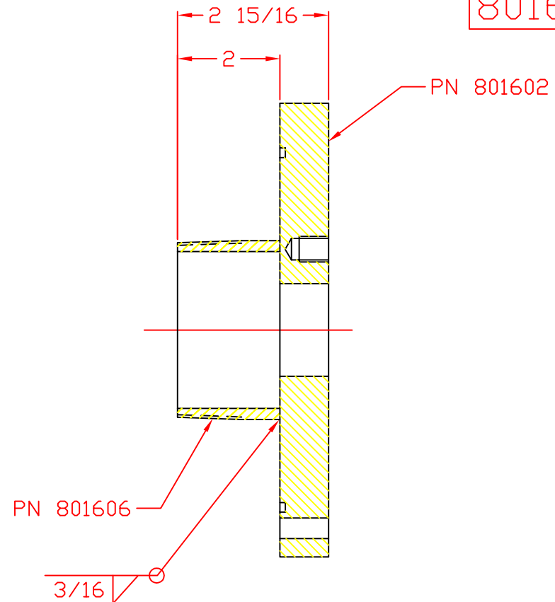
SECTION A-A
