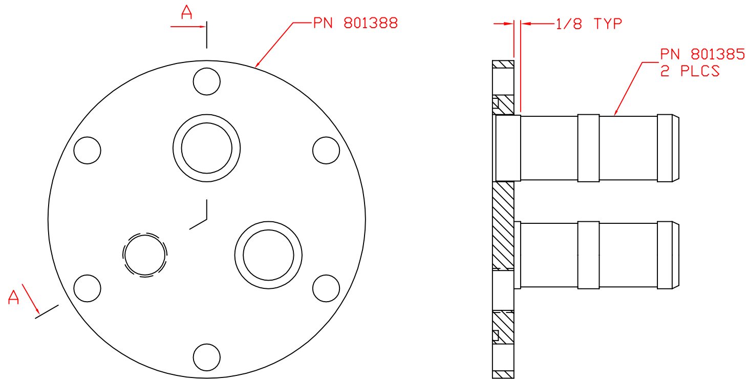
SECTION A-A
